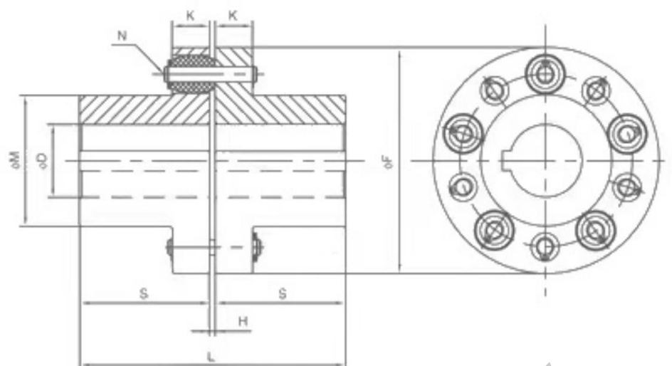
DIN 图纸
