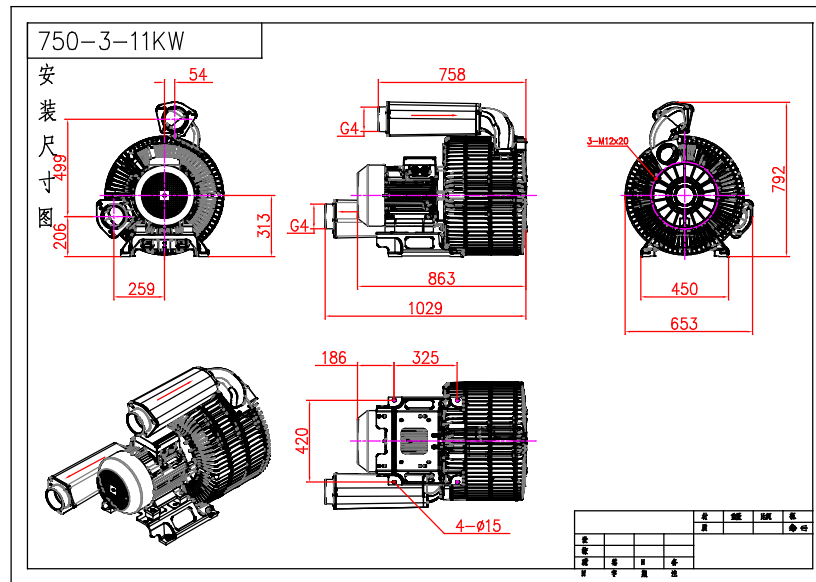
安装尺寸图
