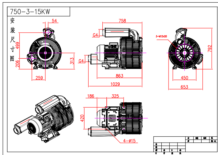
安装尺寸图
