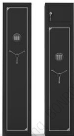
ZXQGH1-2 H1380*W300*D280
