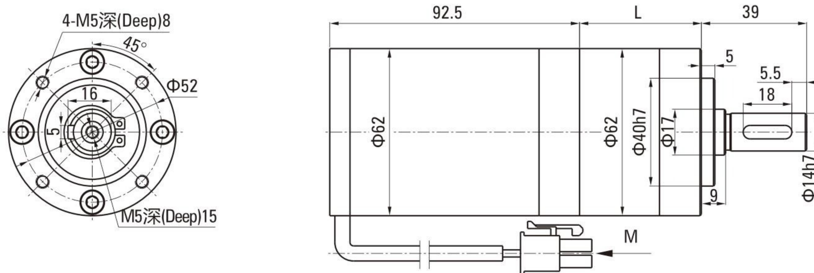
M向视图 (View M)
