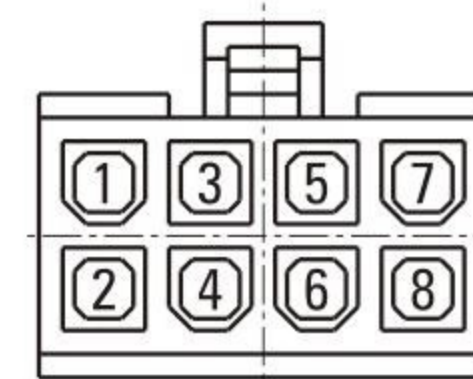
M向视图 (View M)
