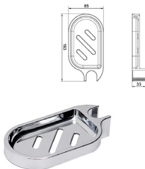
SD05 D19mm D22mm D25mm
