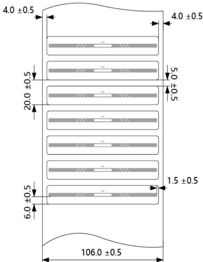
Label 尺寸示意图
