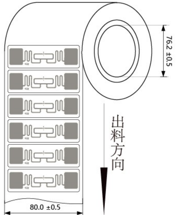
Label 出卷方向示意图
