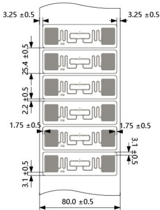
Label 尺寸示意图
