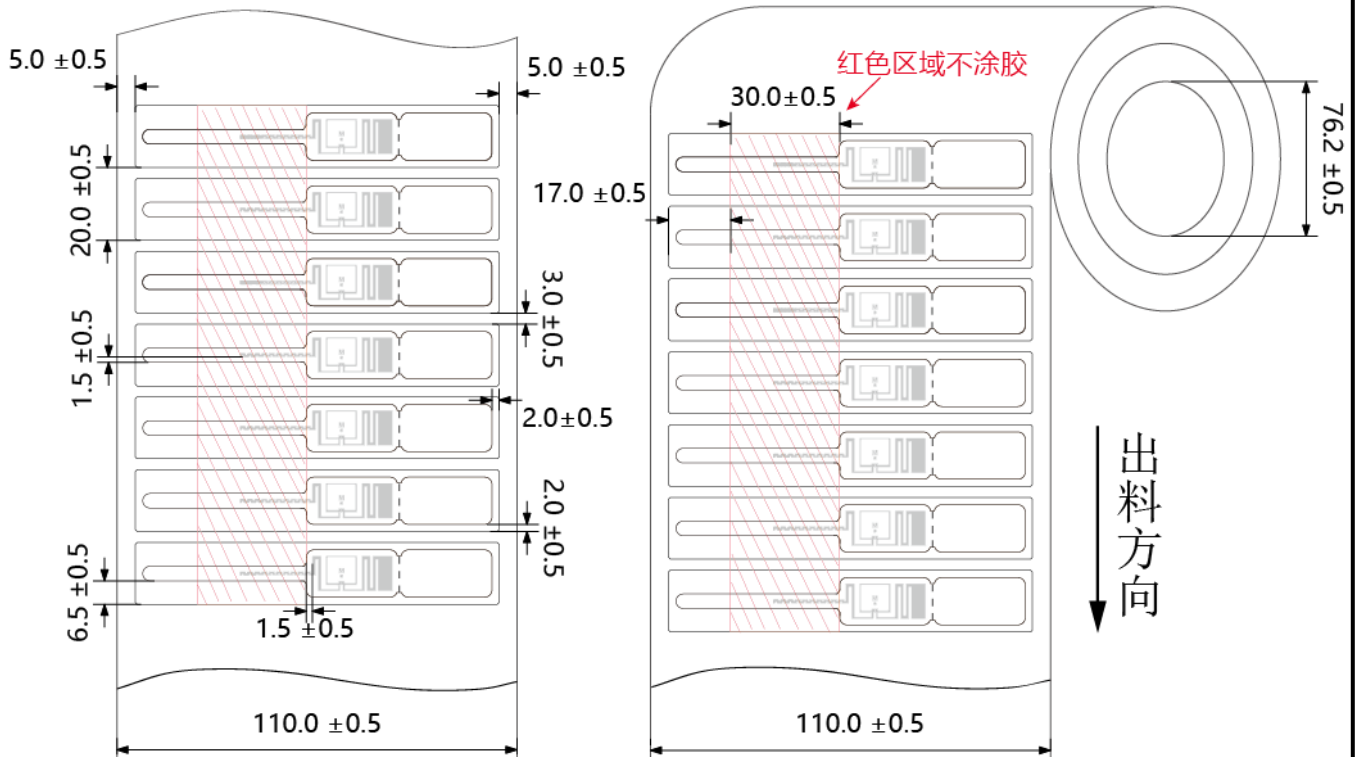
Label 尺寸示意图
