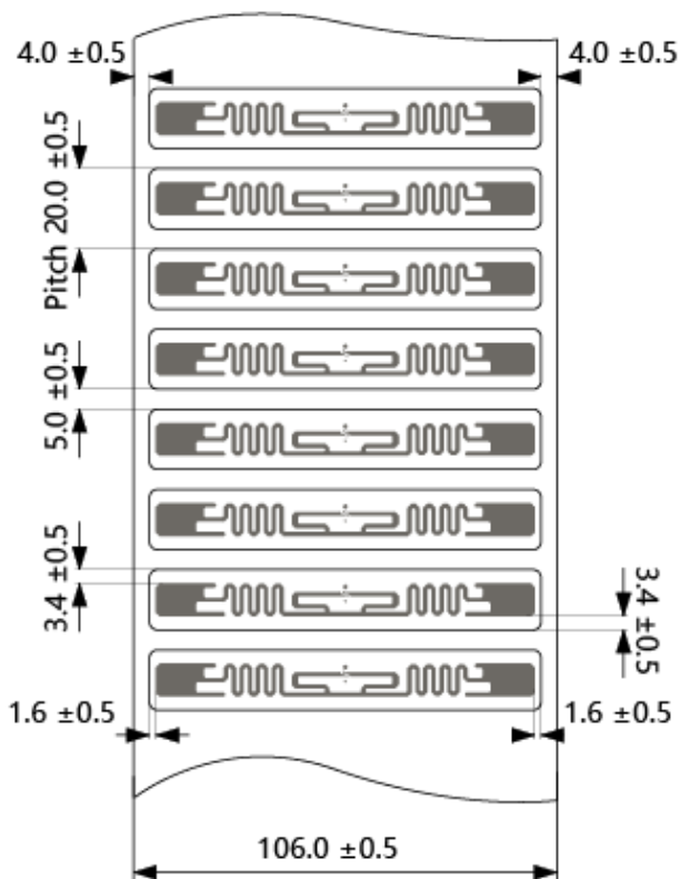
Label 尺寸示意图
