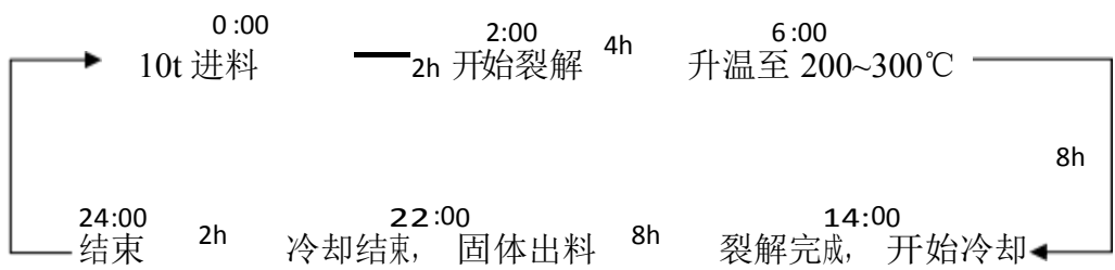
图 1-1 单台设备废轮胎、废塑料、生活垃圾裂解时间节点图
