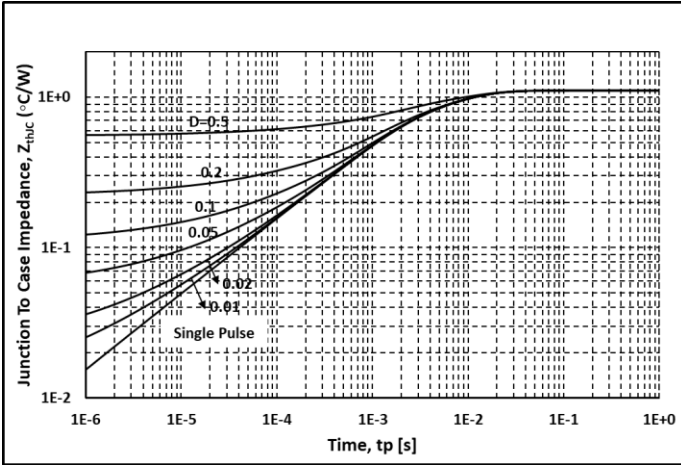
Fig. 25 Thermal impedance
