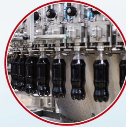
碳酸饮料吹灌旋一体机 CSD Combiblock
