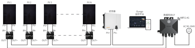
智能优化器连接示意图
